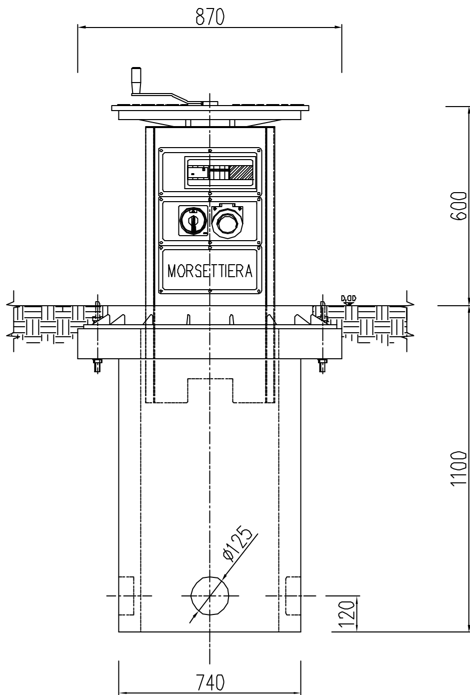
LATO B
